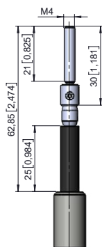
Filetage M4
